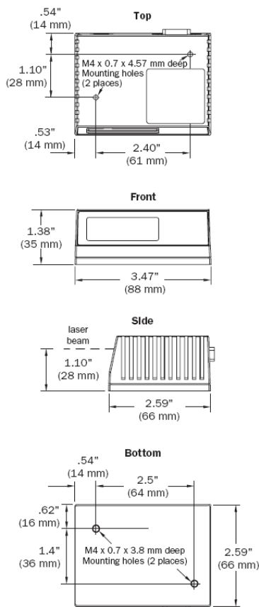
MS-820 Dimensions
