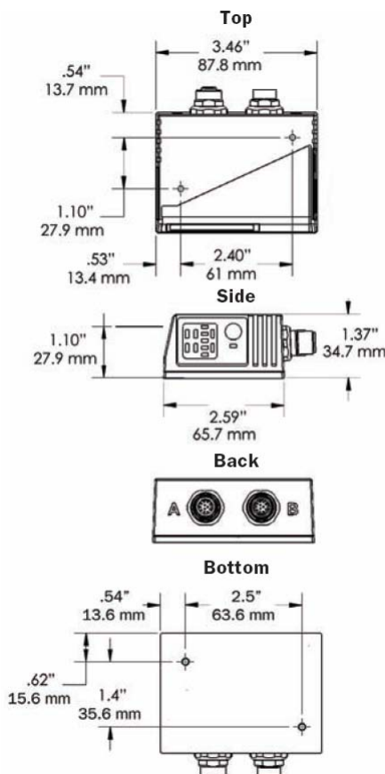
QX-830 Dimensions
